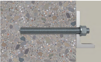
fischer anchor rod FIS A or RGM
