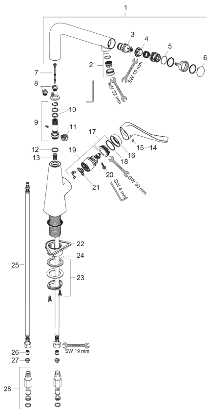
製品分解図
