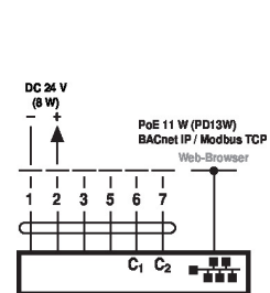
PoE met BACnet IP / Modbus TCP
