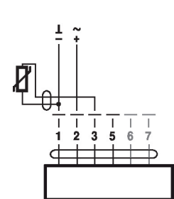
Verbinding met passieve sensor
