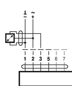
Verbinding met actieve sensor
