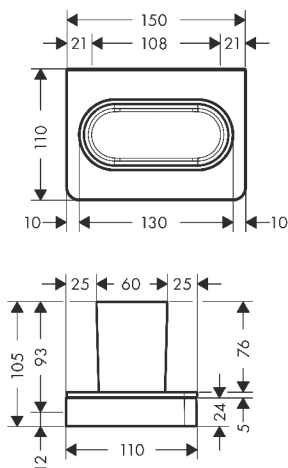
完成図
