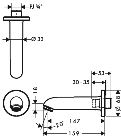
完成図
