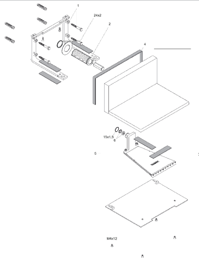
製品分解図
