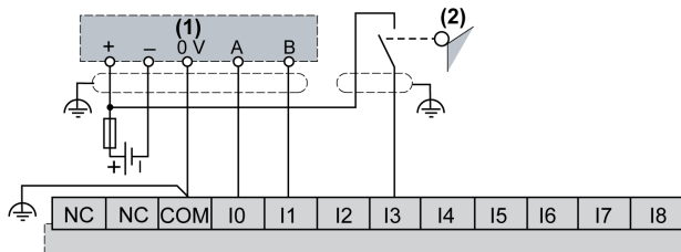
(1) Codificador bifásico sem índice
