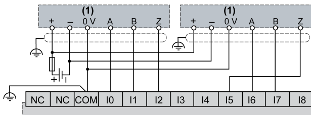
(1) Codificador bifásico com índice
