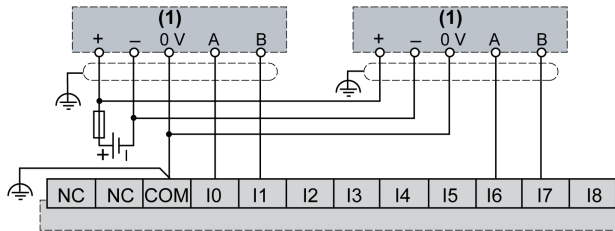
(1) Codificador bifásico sem índice
