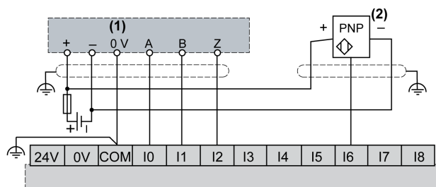
(1) Codificador bifásico com índice
