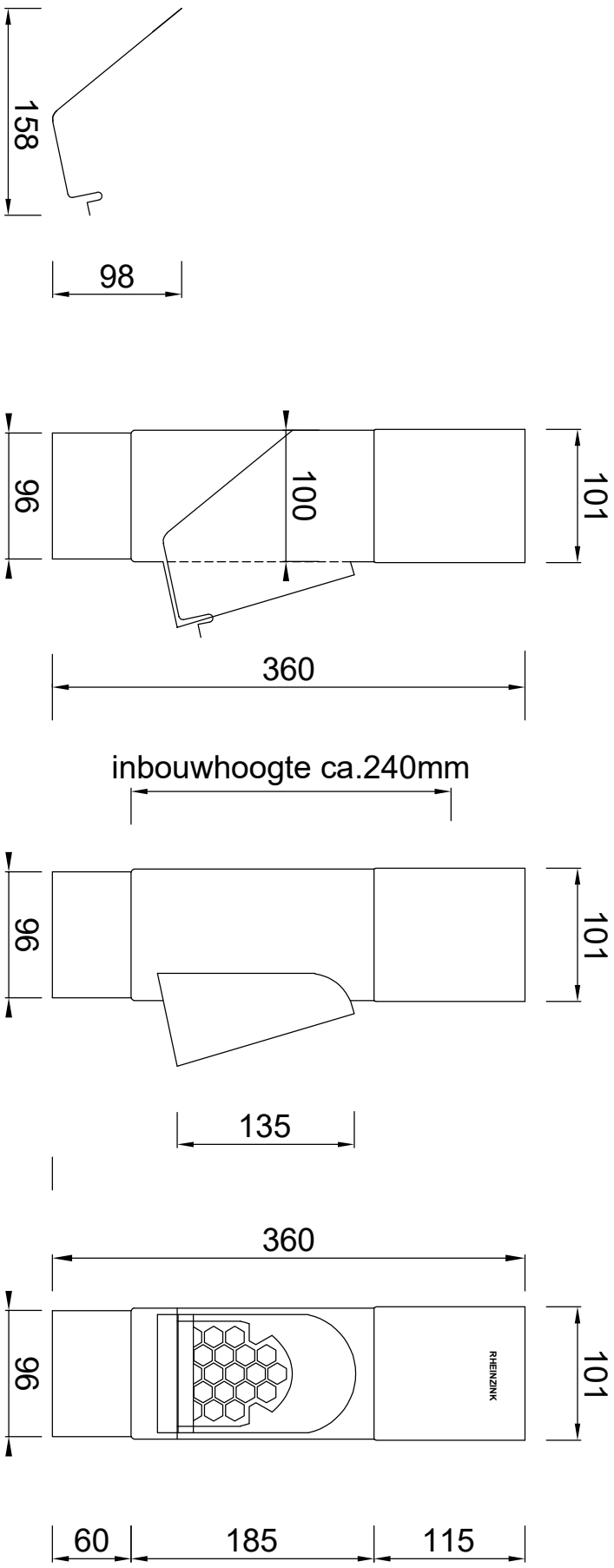
Rooster Zijaanzicht
