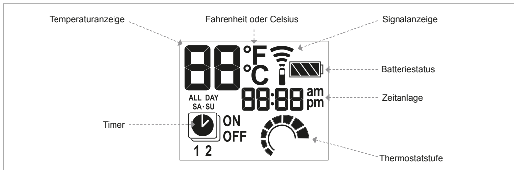
Abb. 18: Display
