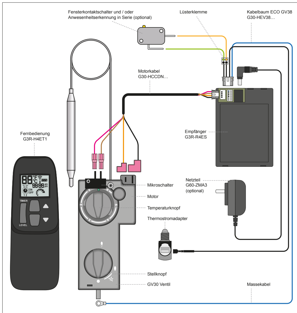
Abb. 20: Anschlussschemata
