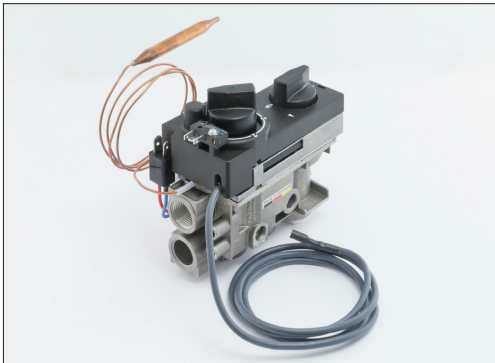
Abb. 1: GV38 Ventil
