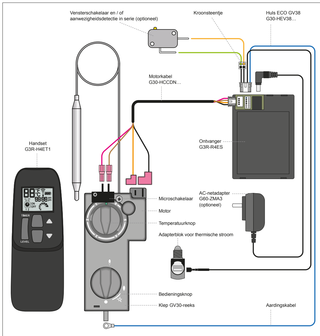
Afb. 20: Bedradingsdiagram
