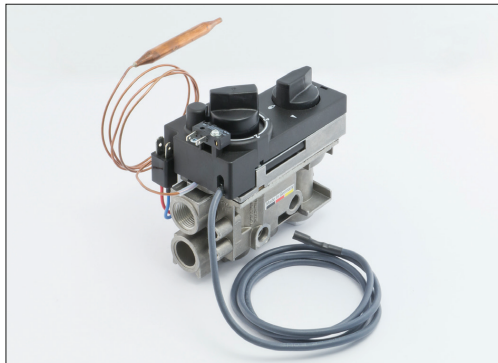
Afb. 1: GV38-klep
