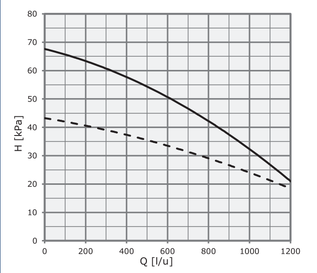
Externe opvoerhoogte boilerpomp
