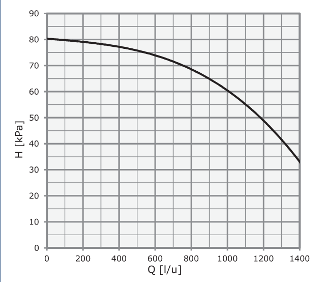
Externe opvoerhoogte cv-pomp koeling
