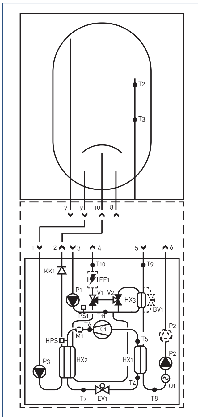
Warmtepomp WPU I-5G + Onderomkasting WPU + voorraadvat WPV
