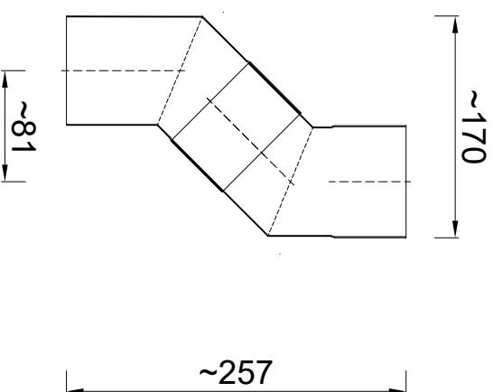
Doorsnede sprong
