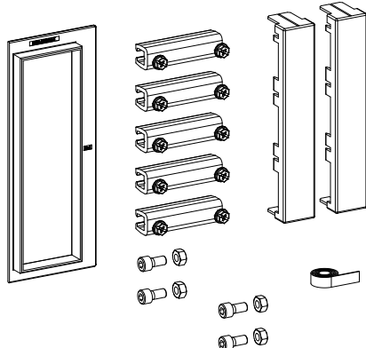
Schrank zu Schrank Verbinder, elektrisch + mechanisch ZSD-SA/SK/VB/5P
