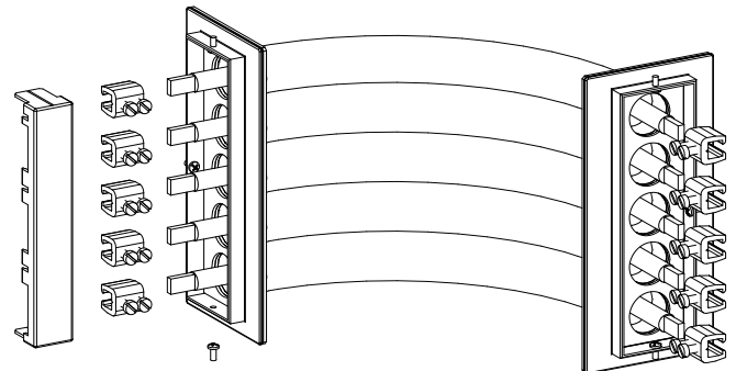
Schrank zu Schrank Eckverbinder ZSD-SA/EV/5P
