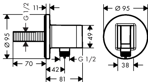
AXOR FixFit Porter Round 36733XX0
