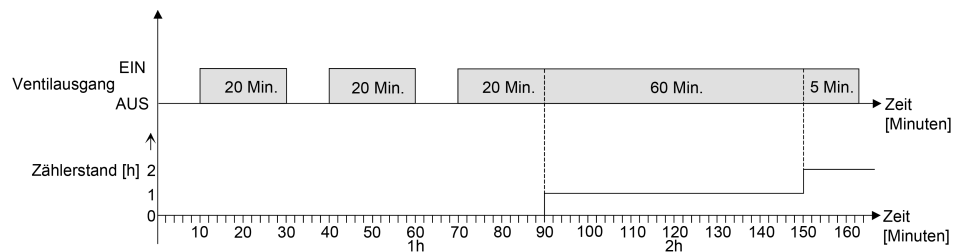
Bild 29: Funktionsweise des Betriebsstundenzählers (am Beispiel eines Vorwärtszählers)
