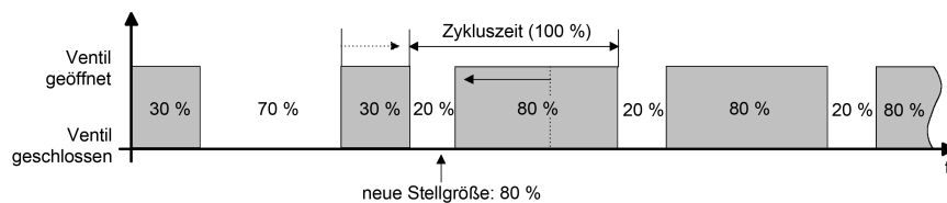
Bild 15: Beispiel einer Stellgrößenänderung 30 % -> 80 % während Schließphase des Ventils
