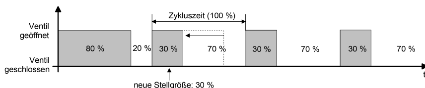
Bild 11: Beispiel einer Stellgrößenänderung 80 % -> 30 % während Öffnungsphase des Ventils
