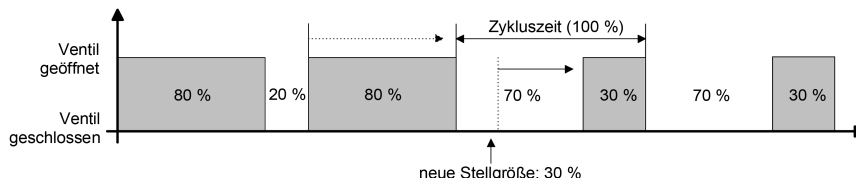
Bild 12: Beispiel einer Stellgrößenänderung 80 % -> 30 % während Schließphase des Ventils
