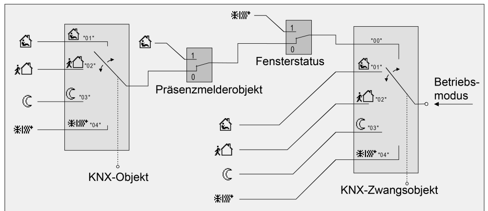
Bild 42: Betriebsmodusumschaltung durch KNX-Objekt mit Präsenzmelder
