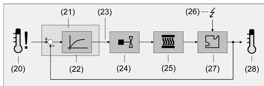
Bild 30: Regelstrecke einer Einzelraum-Temperaturregelung
