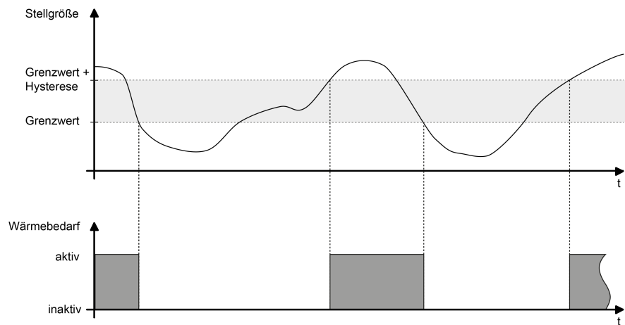
Bild 7: Wärmebedarfsinformation mit beispielhaftem Stellgrößenverlauf
