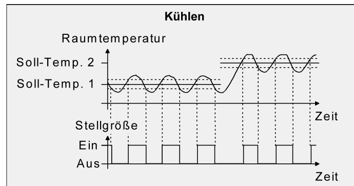
Bild 34: 2-Punkt-Regelung für Einzelbetriebsart "Kühlen"
