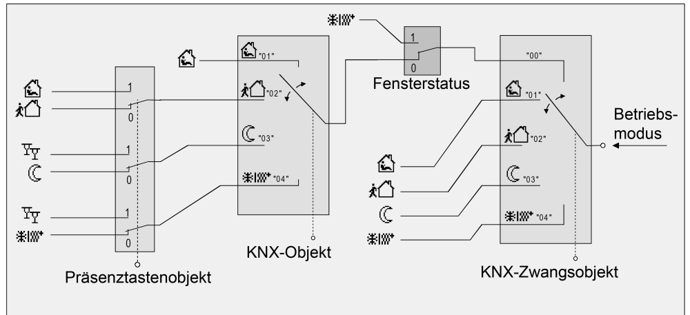
Bild 41: Betriebsmodusumschaltung durch KNX-Objekt mit Präsenztaste
