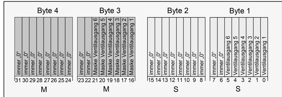
Bild 5: Struktur des Objekts der Sammelrückmeldung
