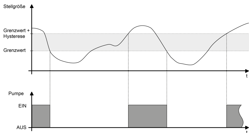
Bild 8: Pumpensteuerung mit beispielhaftem Stellgrößenverlauf
