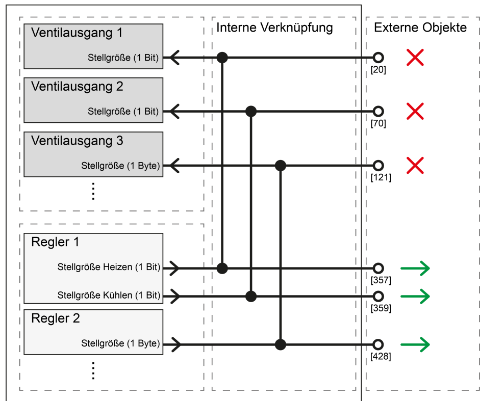
Bild 9: Projektierungsbeispiel zur internen Gruppenkommunikation
