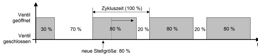
Bild 14: Beispiel einer Stellgrößenänderung 30 % -> 80 % während Öffnungsphase des Ventils
