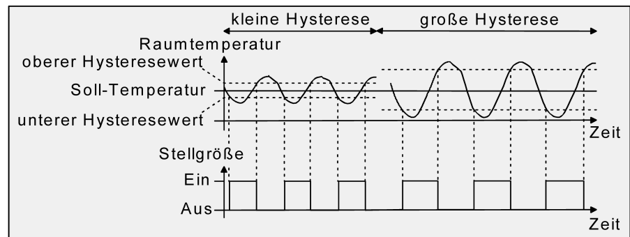
Bild 38: Auswirkungen der Hysterese auf das Schaltverhalten der Stellgröße einer 2-Punkt-Regelung
