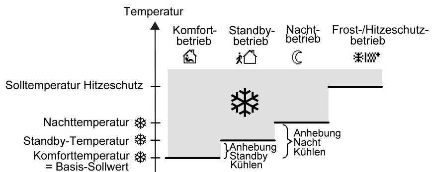
Bild 45: Solltemperaturen in der Betriebsart "Kühlen"
