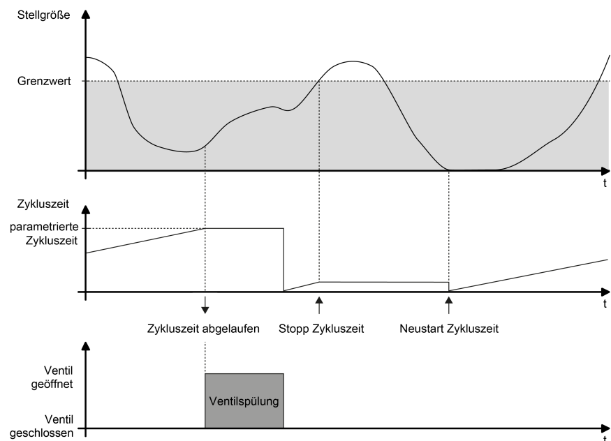
Bild 28: Beispiel eines minimalen Stellgrößen-Grenzwerts für die intelligente Ventilspülung
