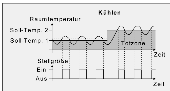
Bild 36: 2-Punkt-Regelung für Mischbetriebsart "Heizen und Kühlen" bei aktivem Kühlbetrieb
