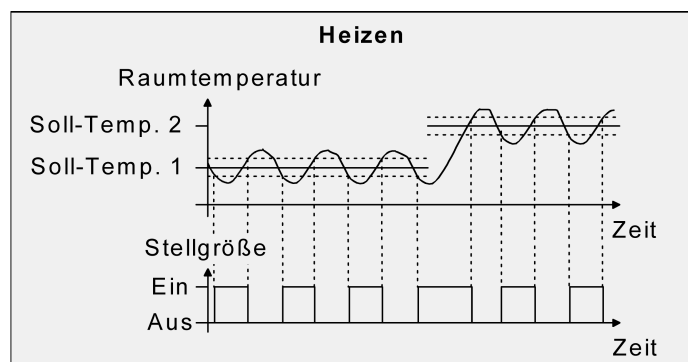
Bild 33: 2-Punkt-Regelung für Einzelbetriebsart "Heizen"
