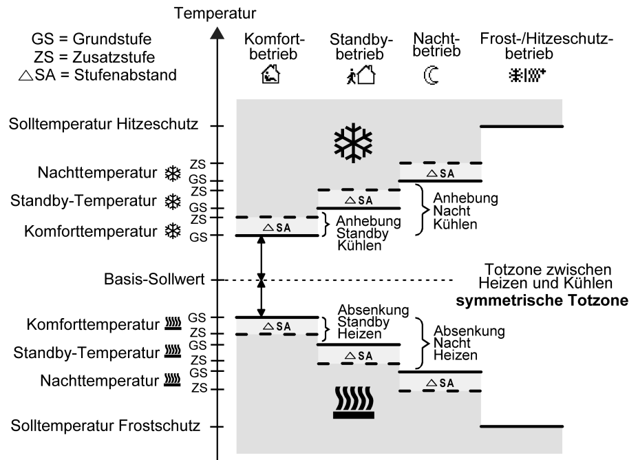
Bild 49: Solltemperaturen in der Betriebsart "Grund- und Zusatzheizen und -kühlen" mit symmetrischer Totzone
