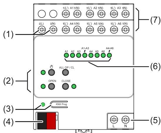
Bild 1: Geräteaufbau
