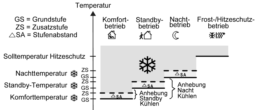
Bild 46: Solltemperaturen in der Betriebsart "Grund- und Zusatzkühlen"
