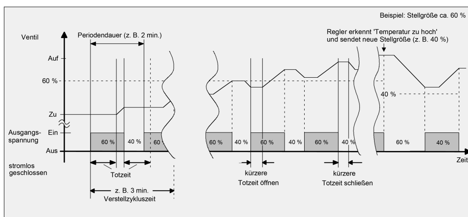
Bild 19: Idealisierter Verlauf des Ventilhubes exemplarisch dargestellt für eine Zykluszeit < Verstellzykluszeit
