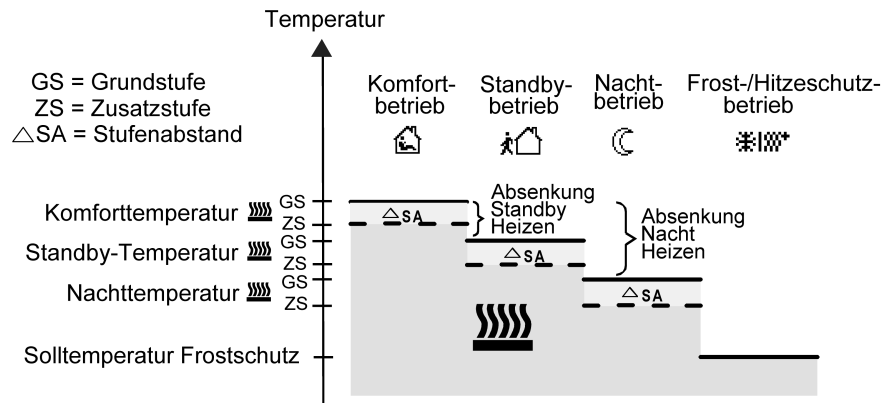
Bild 44: Solltemperaturen in der Betriebsart "Grund- und Zusatzheizen"
