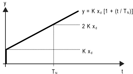
Bild 37: Funktion der Stellgröße einer PI-Regelung
