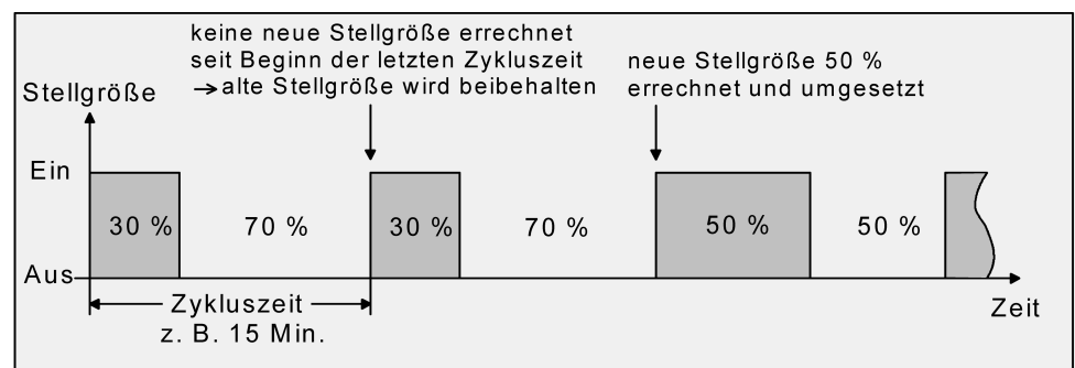
Bild 32: Schaltende PI-Regelung
