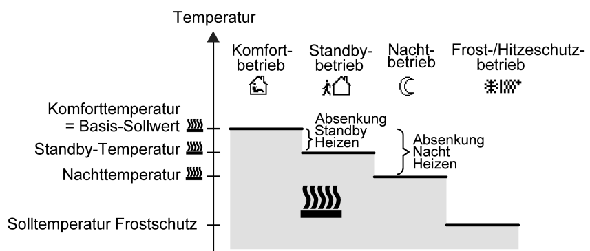
Bild 43: Solltemperaturen in der Betriebsart "Heizen"
