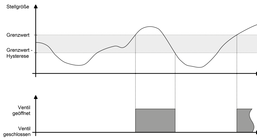
Bild 17: Beispiel einer Stellgrößenauswertung mit Grenzwert
