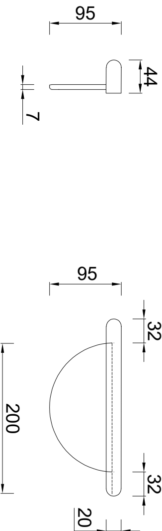
Voor-aanzicht
