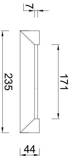
Bovenaanzicht
