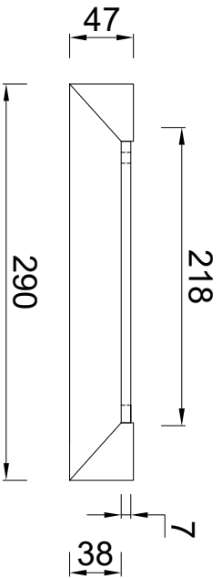
Bovenaanzicht links
