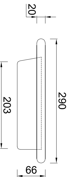
Zijaanzicht rechts
