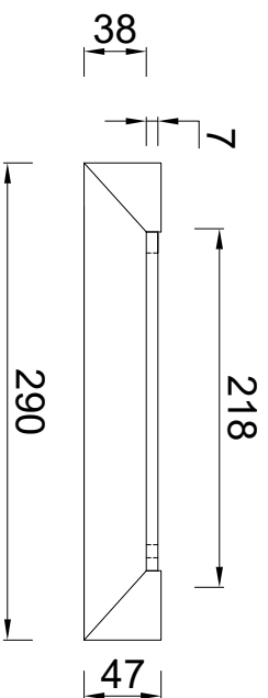
Bovenaanzicht rechts
