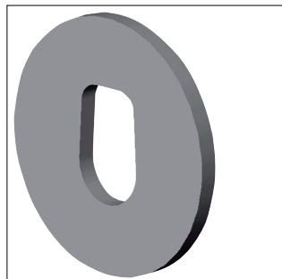
Klemplaat voor hamerkopbout M8 (4 stuks)
