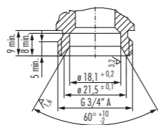
Lösbare Verbindung mit Rohraußengewinde und Gewindefreistich
