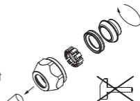
Klemmverschraubung MKV-M
