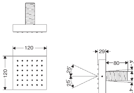
完成図
