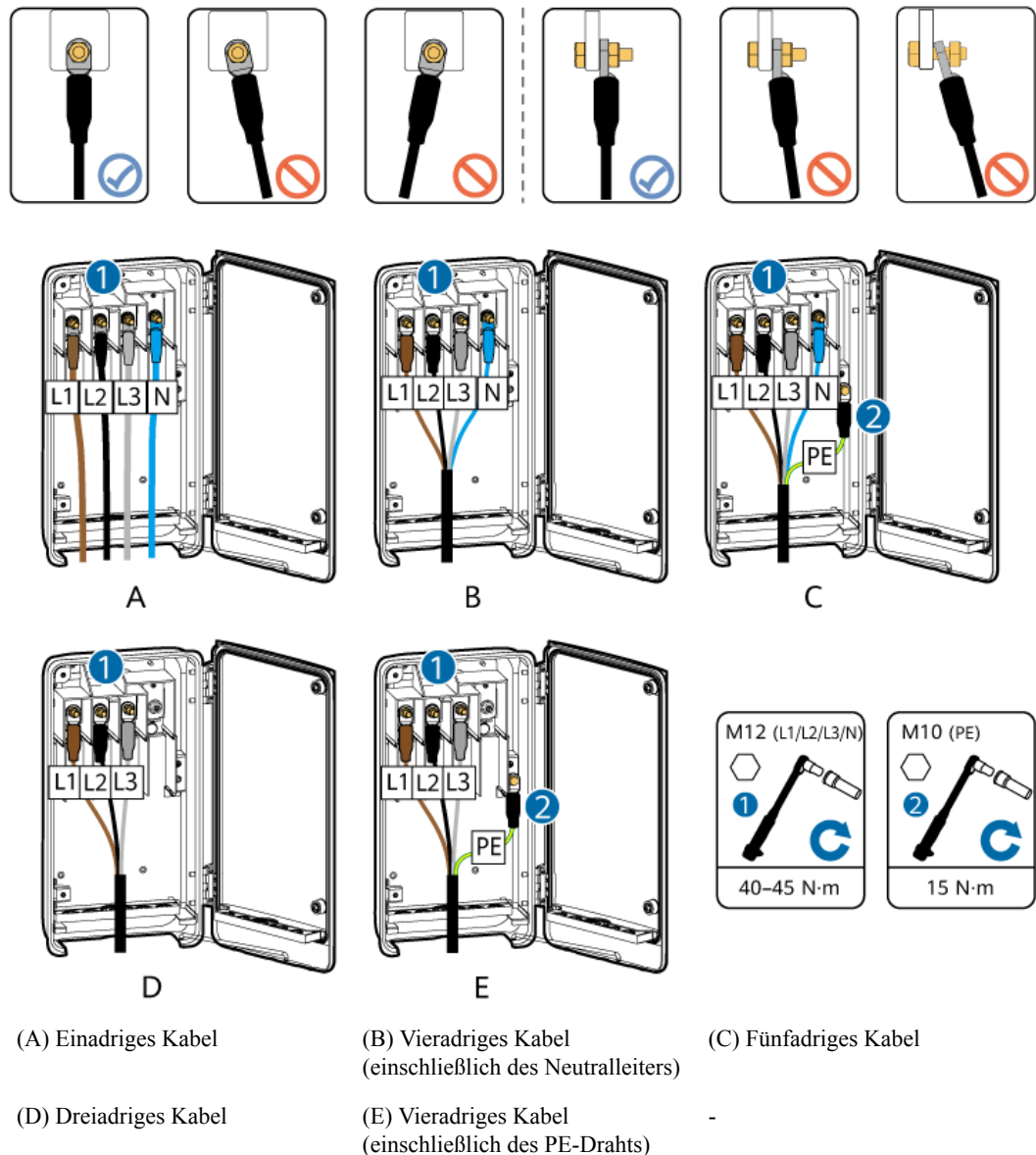
Abbildung 5-6 Kabelverbindung
