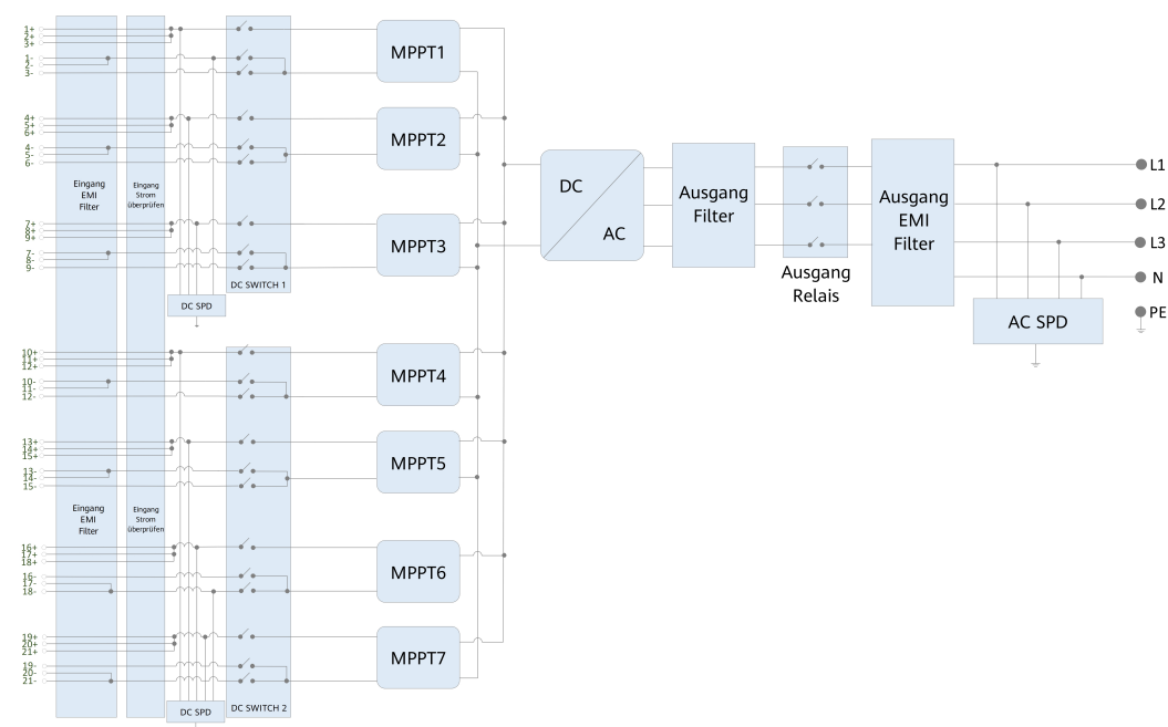
Abbildung 2-9 Stromlaufplan
