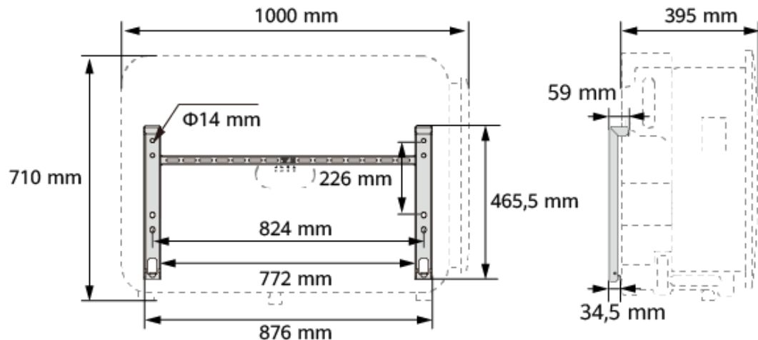
Abbildung 4-2 Abmessungen
