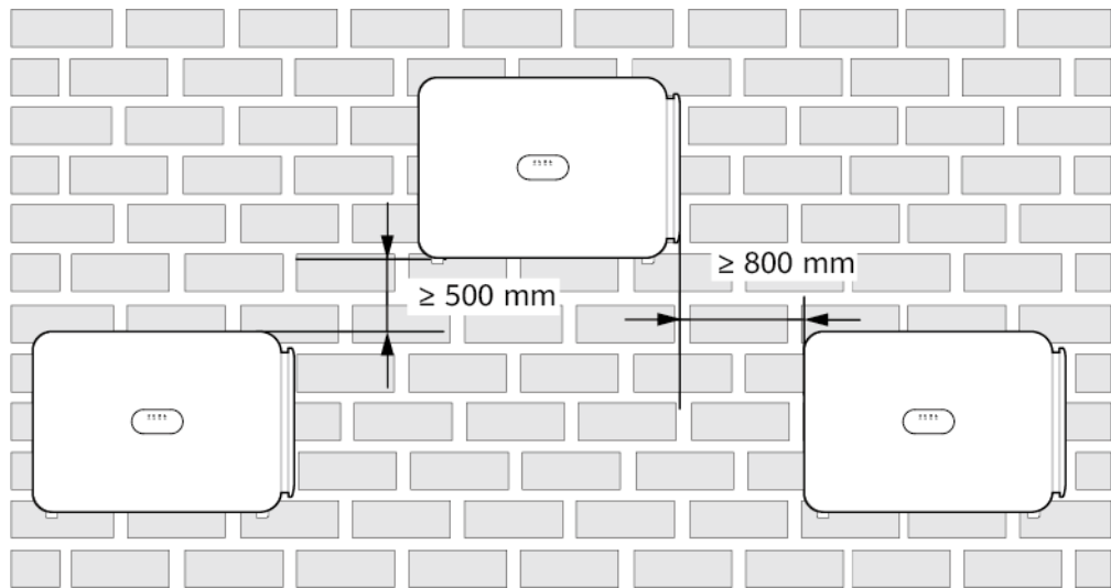
Abbildung 4-5 Dreiecks-Montagemethode (empfohlen)
