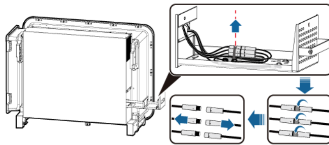
Abbildung 8-3 Trennen der Kabel
