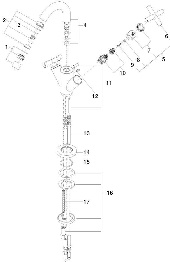
18 Ablaufgarnitur 04.11.01.001.00-ff
