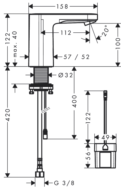
Maattekening
