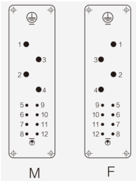
Pinbelegung
