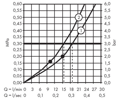
AXOR 300 2jet 35303XX0
