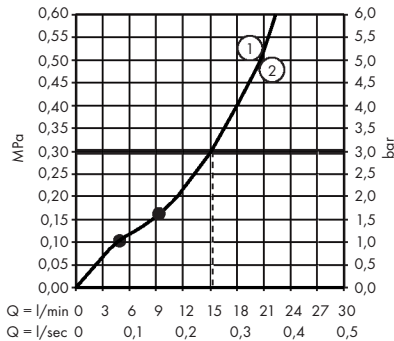
AXOR 250 2jet 35296XX0
