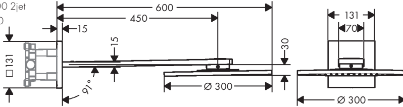
AXOR 250/250 2jet 35310XX0
