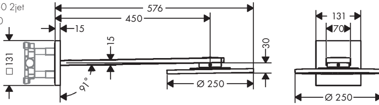
AXOR 300 2jet 35303XX0
