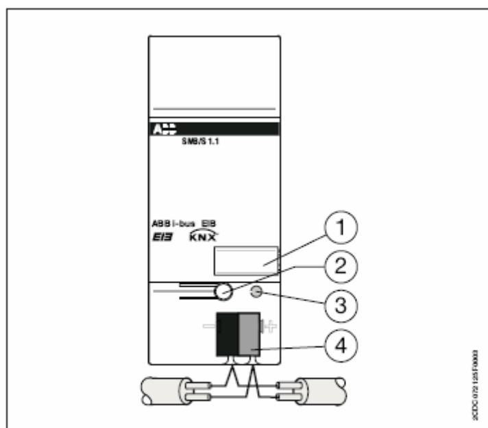
Abb. 2: Anschlussbild SMB/S 1.1
