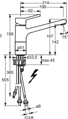
HANSAFORM 4912 1103
