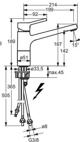
HANSAFORM 4912 1103
