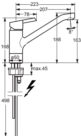
HANSAPINTO 4538 1173
