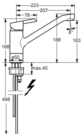
HANSAPINTO 4538 1173
