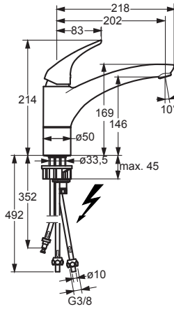
HANSATWIST 0912 1183 0912 1185
