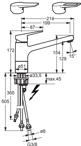
HANSATWIST 0912 1183 0912 1185
