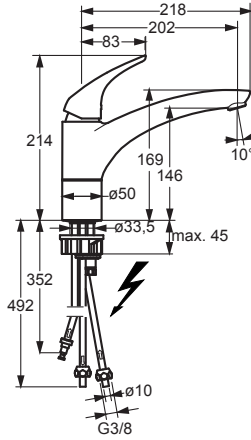
HANSATWIST 0912 1183 0912 1185
