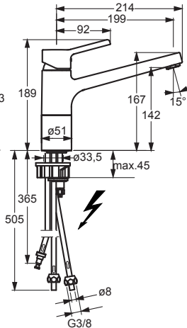
HANSAFORM 4912 1103
