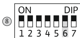
Fig. 17: Микропереключатель 1: Pump Kick
