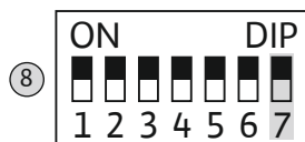
Fig. 16: Микропереключатель 1: внутренний зуммер
