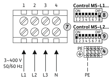
Fig. 7: Подключение к сети 3~400 В без главного выключателя
