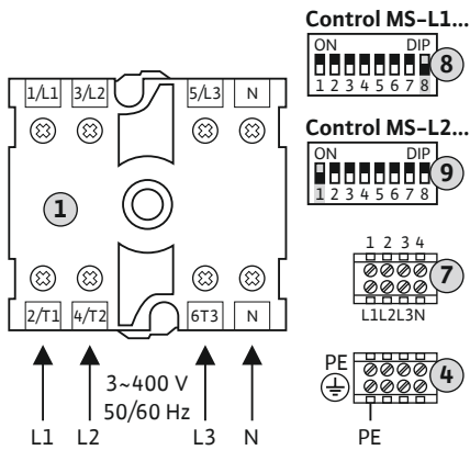
Fig. 5: Подключение к сети 3~400 В с главным выключателем
