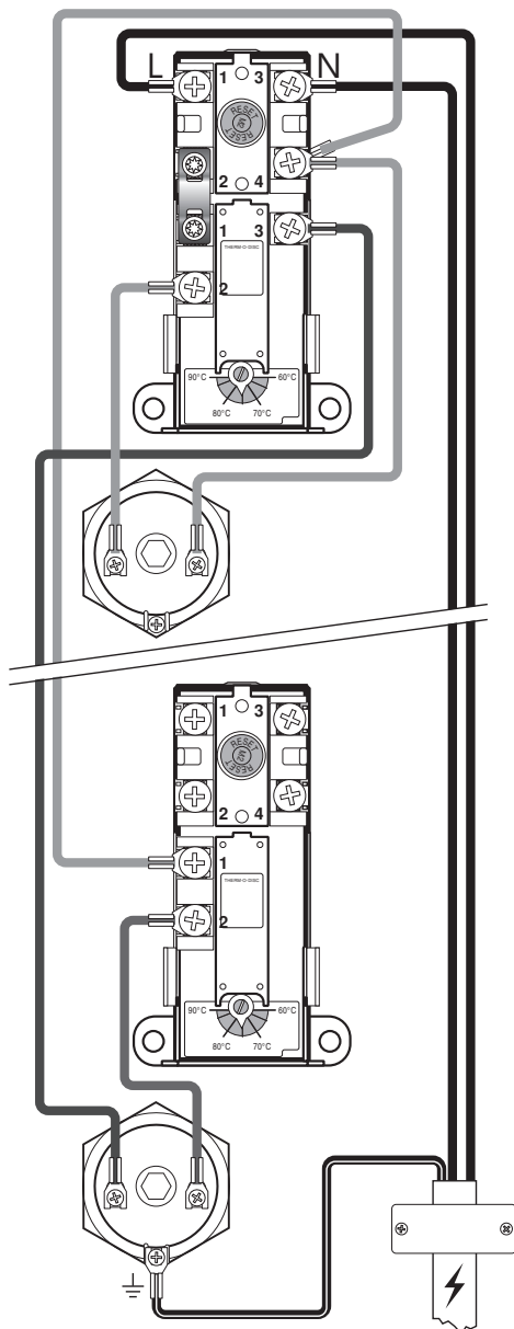
Elektrische aansluiting, schematisch 4,5+4,5 kW
