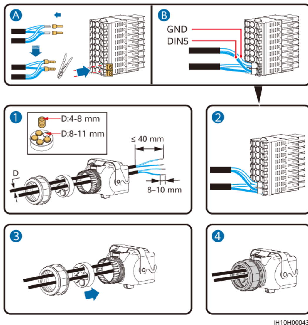
Afbeelding5-39 Kabels installeren
