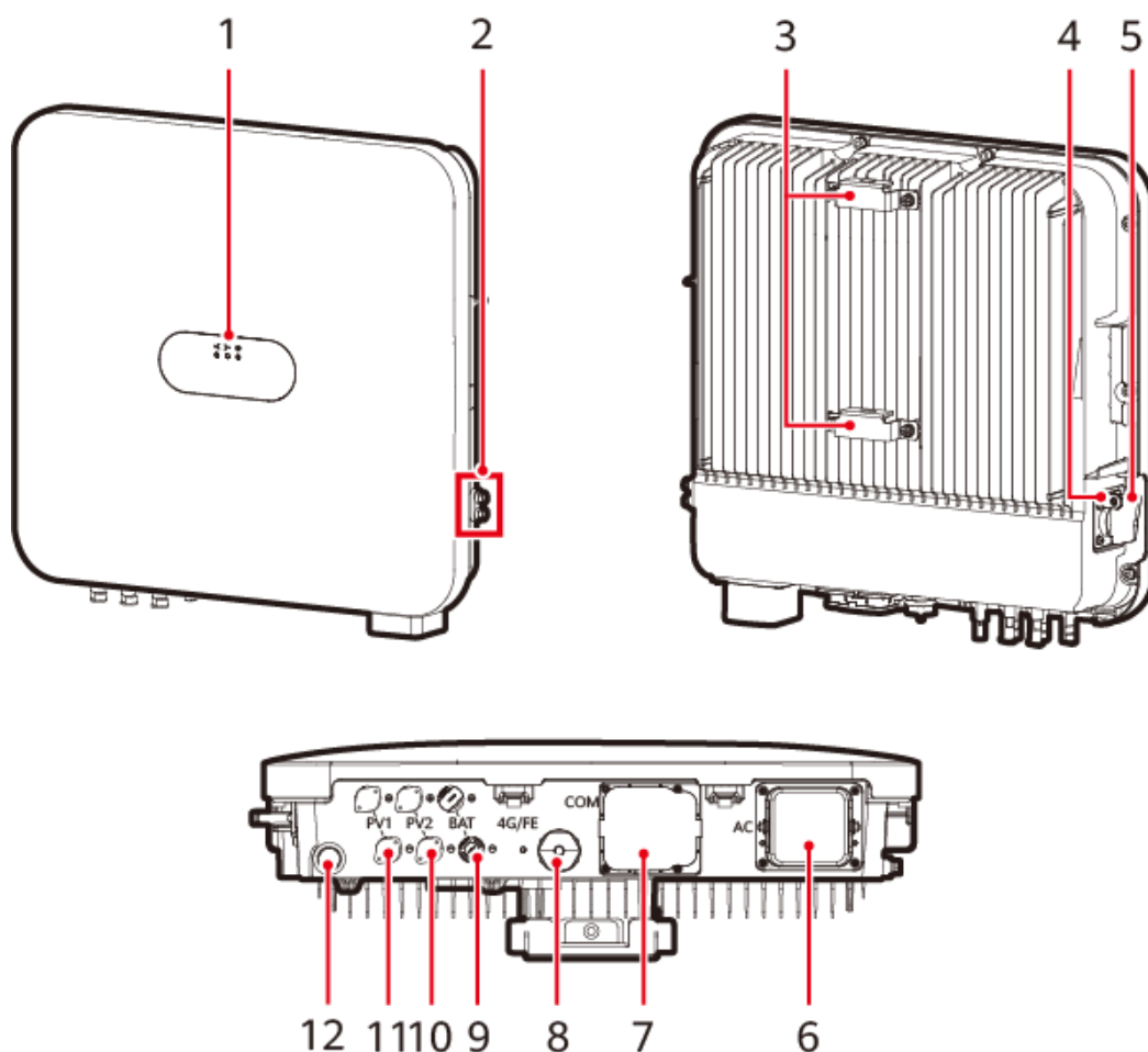
Afbeelding2-7 Uiterlijke kenmerken
