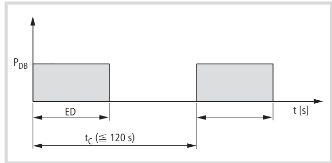
рисунок 121: Продолжительность включения
