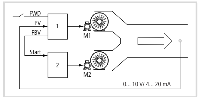
рисунок 91: Блок-схема, вентиляция с „двухступенчатым регулированием“
