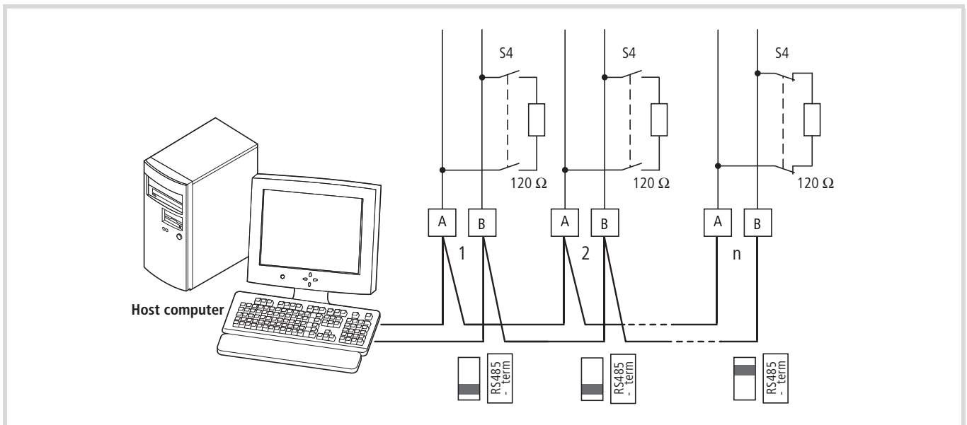
рисунок 106: Сеть Modbus с M-Max™
