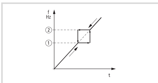
рисунок 83: Диапазон заданного значения для скрытия частоты
