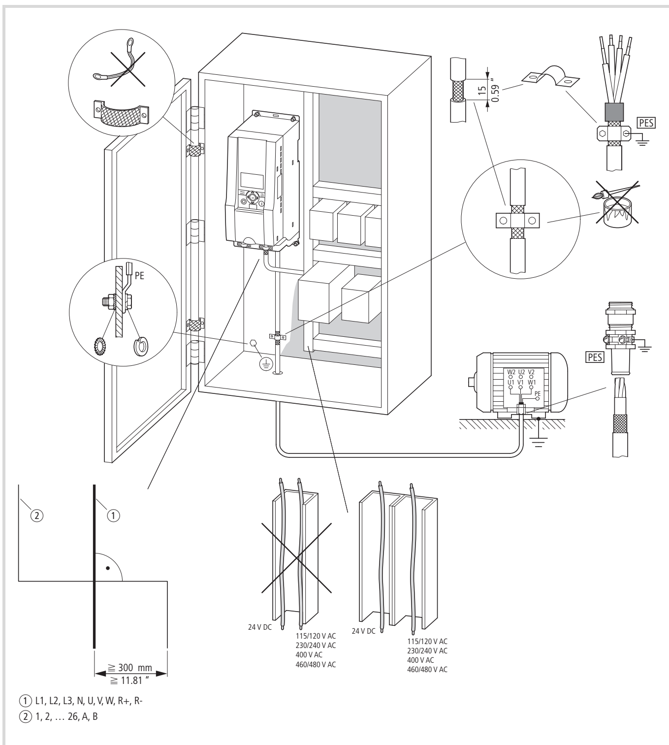
рисунок 26: Монтаж с соблюдением требований ЭМС (пример: M-Max™)
