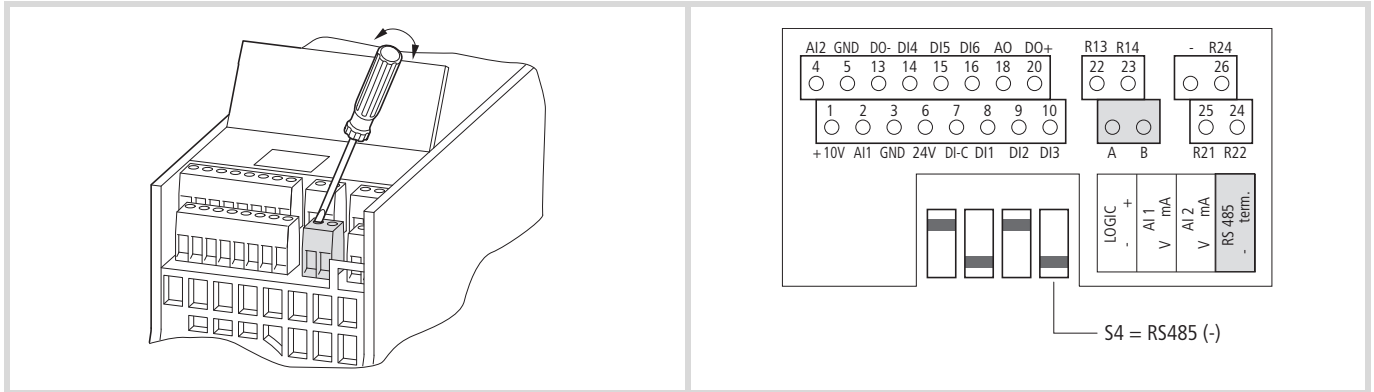
рисунк 52:Соединительные клеммы последовательного интерфейса и микровыключатель S4 (оконечная нагрузка шины)
