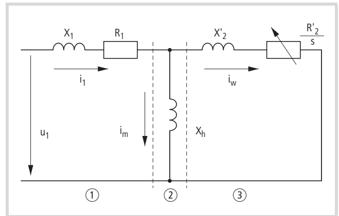
рисунок 99:Заменяющая электрическая схема трехфазного асинхронного двигателя
