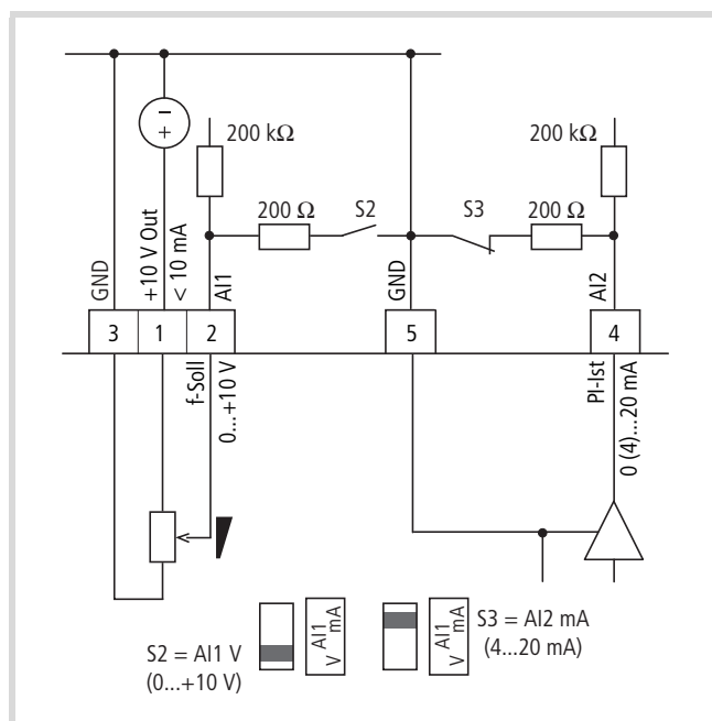
рисунок 41: Аналоговые входы заданных значений AI1 и AI2 Пример подключения: Потенциометр (4,7 кОм) M22-R4K7; арт. № 229490
