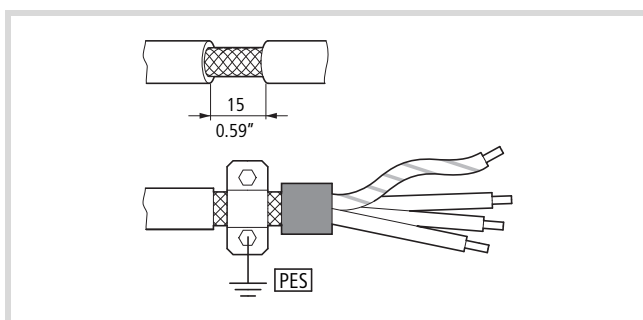
рисунок 31: Экранированная соединительная линия
