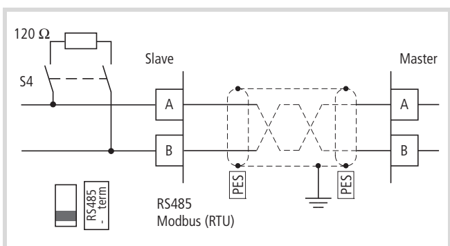
рисунк 53:Подключение двухпроводной линией RS485 (подчиненное устройство = преобразователь частоты M-Max™)
