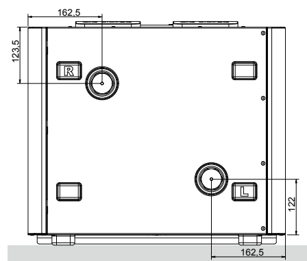
Onderaanzicht
