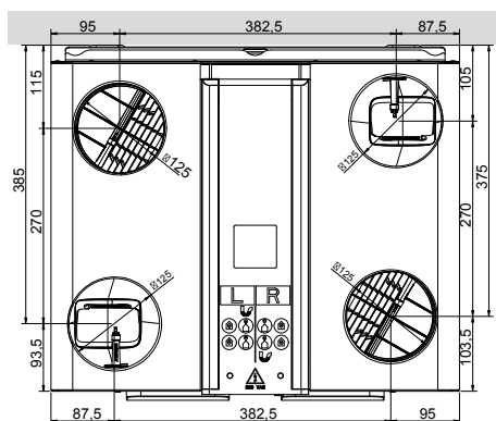
Bovenaanzicht
