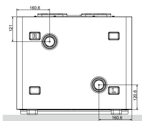
Onderaanzicht
