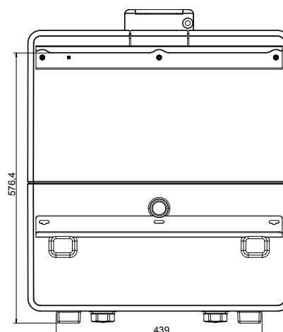
Achteraanzicht
