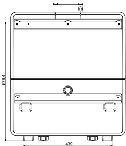
Vue arrière
