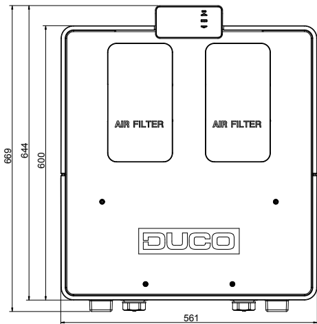
Vue avant
