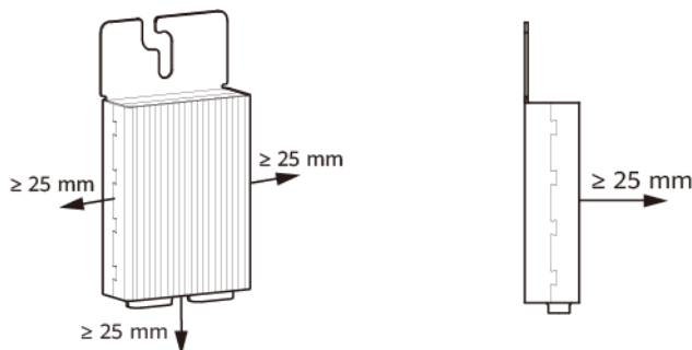
Afbeelding3-1 Spelingsvereisten
