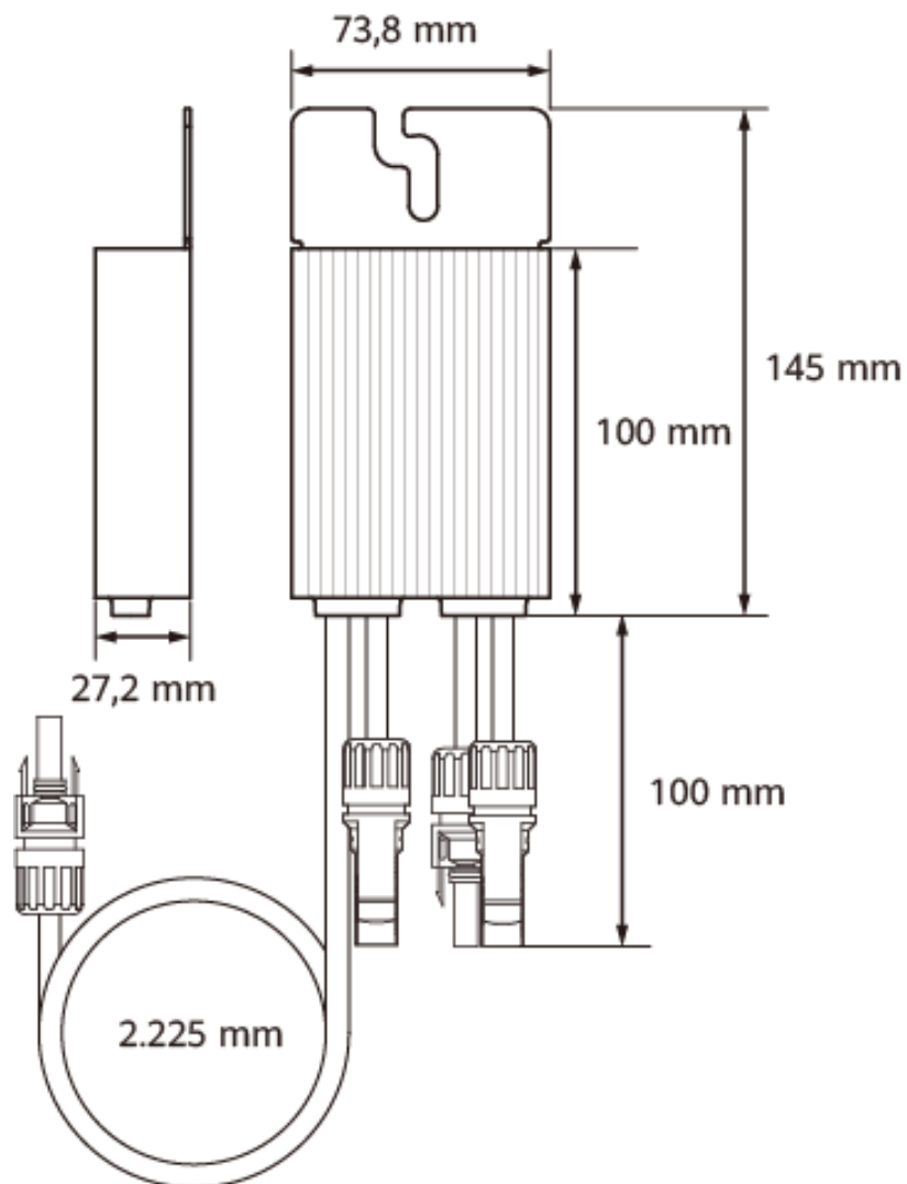
Afbeelding2-3 Afmetingen MERC-600W-PA0
