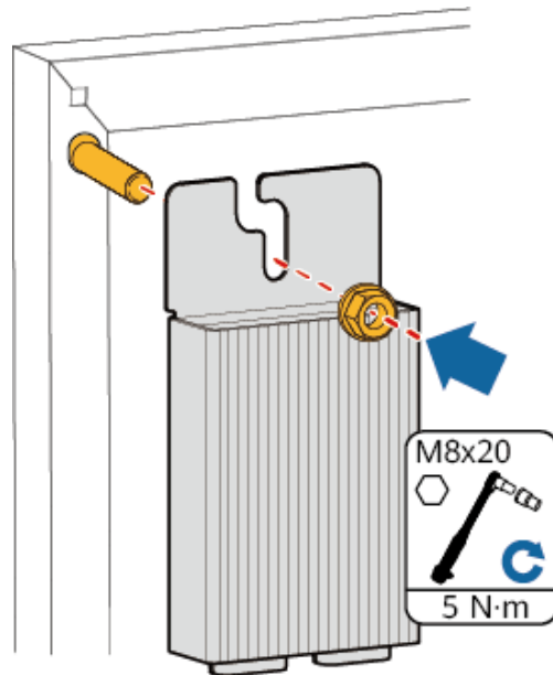
Afbeelding3-4 De optimizer installeren op het frame voor de PV-module met een boutconstructie
