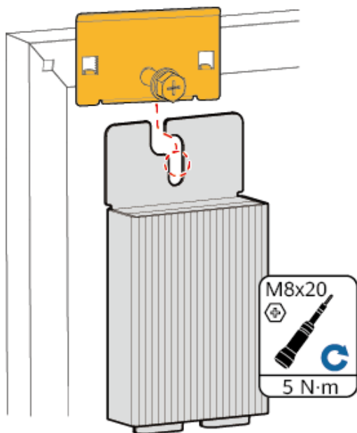
Afbeelding3-5 De optimizer installeren op het frame voor de PV-module met een framemontagesteun (installatie aan voorkant)
