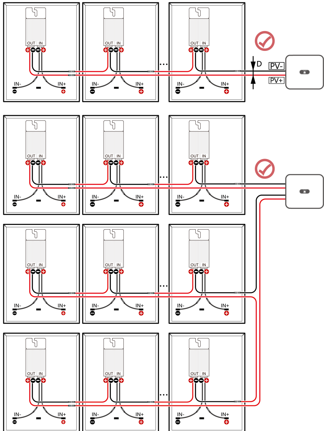
Afbeelding3-7 Vereiste bekabeling
