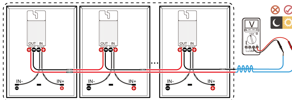
Afbeelding3-6 De spanning van de PV-reeks meten
