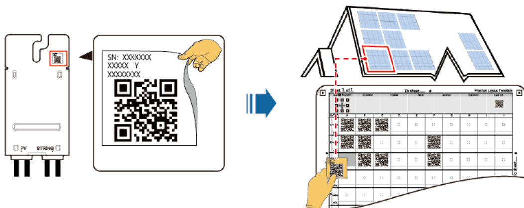
Afbeelding3-2 Het label verwijderen en op de fysieke lay-outsjabloon bevestigen
