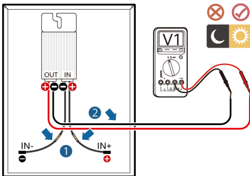
Afbeelding6-1 De spanning van een optimizer meten
