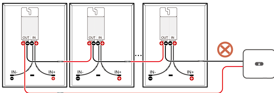
Afbeelding3-8 Verboden bekabeling
