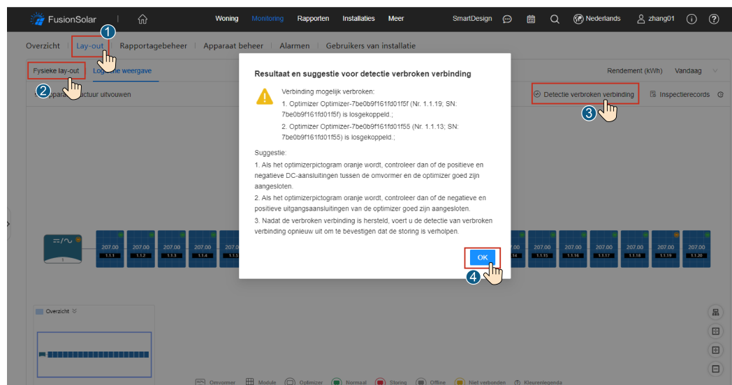
Afbeelding4-2 Detectie verbroken verbinding optimizer
