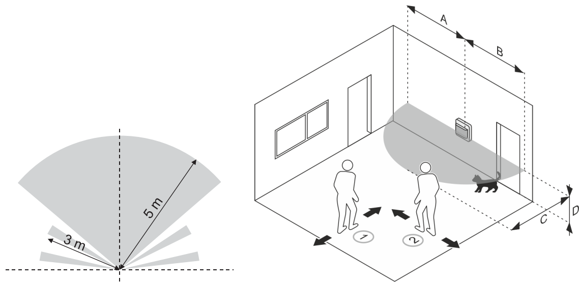
Abb. 16: Erfassungsbereiche flex Bedienelement
