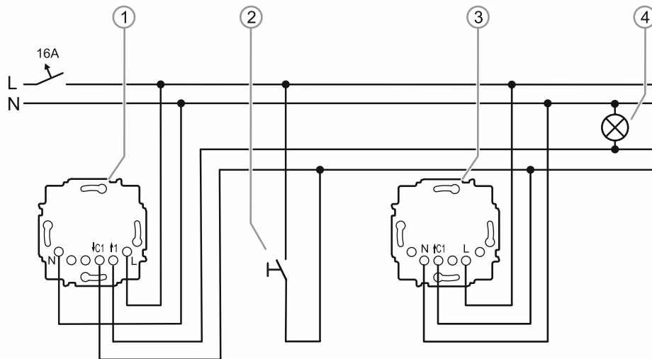
Abb. 32: Anwendungsbeispiel: Korridor mit hellen und dunklen Bereichen – Anschluss
