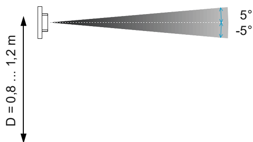
Abb. 10: Öffnungswinkel 64762-xxx
