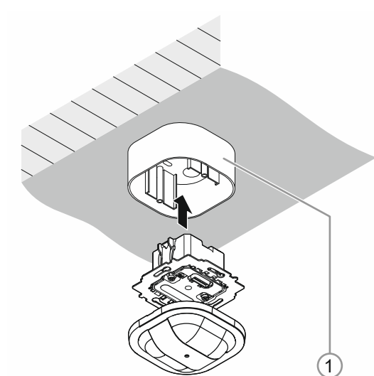
Abb. 2: Oberflächenmontage Busch-flexTronics®
