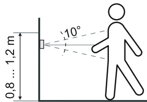
Abb. 15: Öffnungswinkel flex Bedienelement
