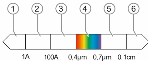
Abb. 22: Funktionsprinzip IR-Sensorik
