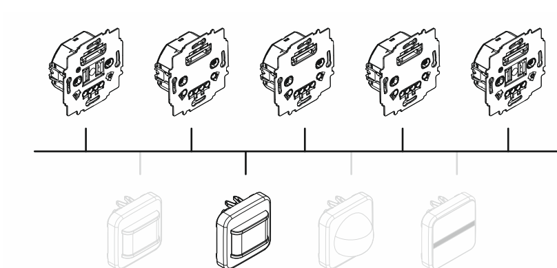
Abb. 7: 180 flex, Komfort Sensor mit Selectlinse: Funktionen in Kombination mit UP-Einsätzen
