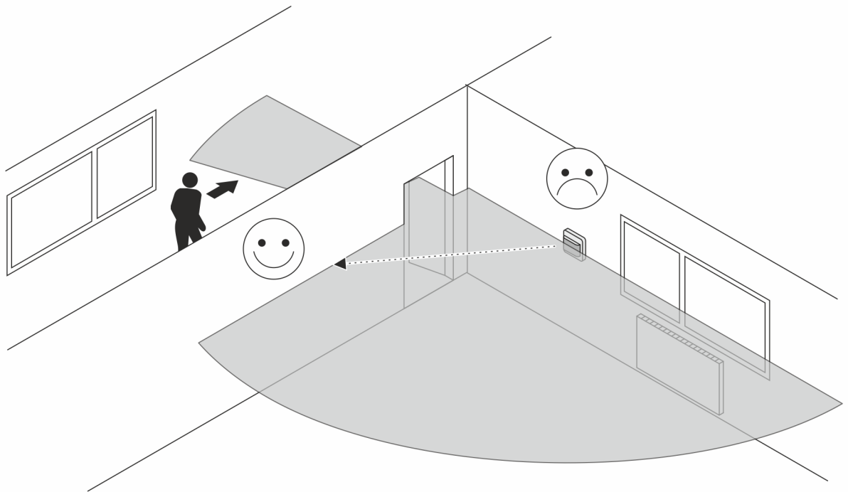
Abb. 36: Störquelle Bewegungsmelder: Geöffnete Tür
