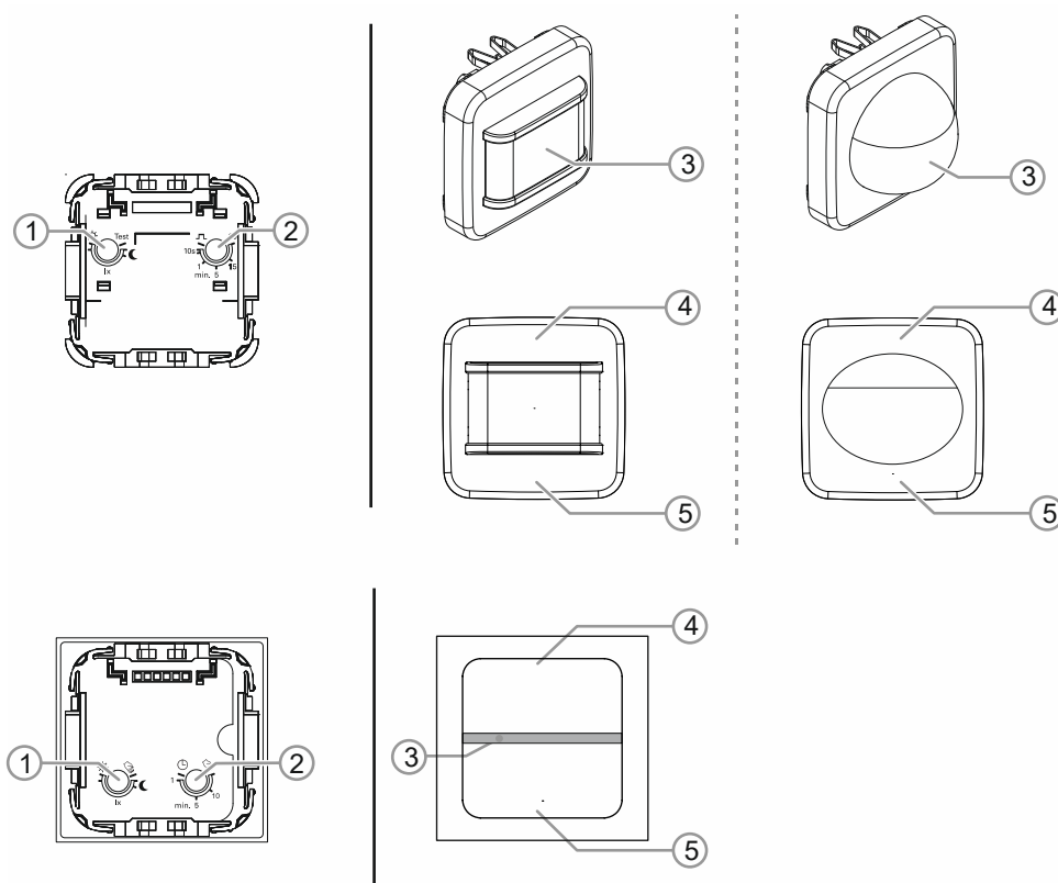
Abb. 19: Bedienelemente
