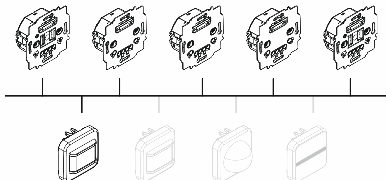
Abb. 6: 180 flex, Basic Sensor mit Selectlinse: Funktionen in Kombination mit UP-Einsätzen
