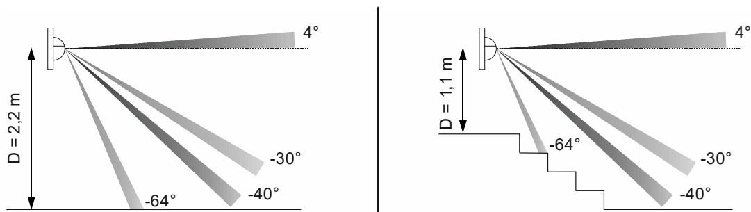
Abb. 13: Öffnungswinkel 64764-xxx
