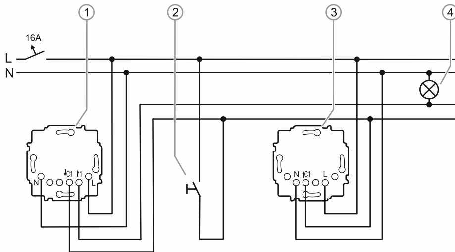
Abb. 17: Anschlussbeispiel: Hauptgerät (Main) mit Nebengerät (Sub) und Nebenstelle
