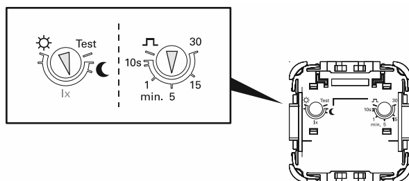
Abb. 3: Einstellung über Trimmer: Sensoren
