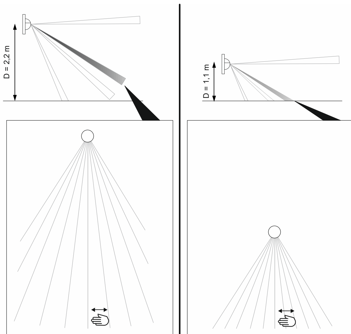
Abb. 29: Montagehöhen
