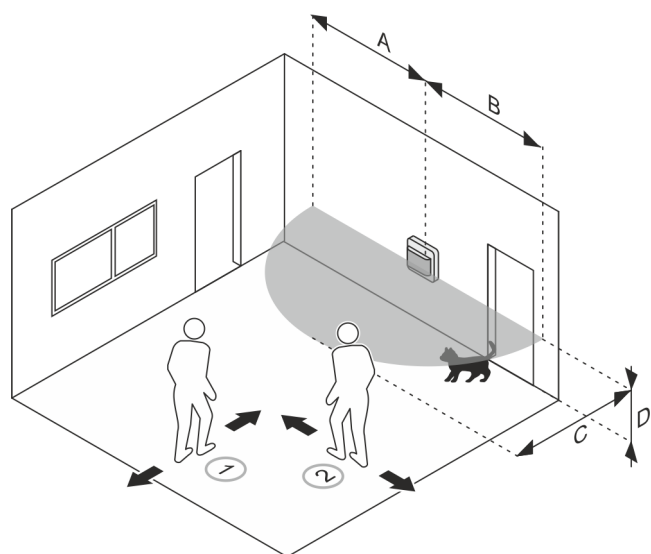
Abb. 11: Erfassungsbereiche: Prinzip 64762-xxx
