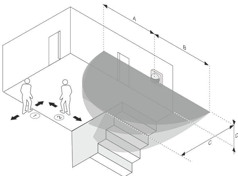
Abb. 14: Erfassungsbereiche: Prinzip 64764-xxx
