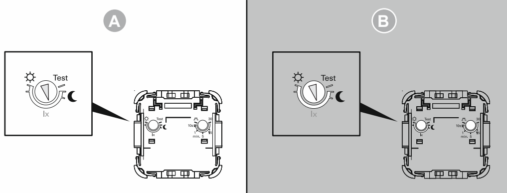
Abb. 31: Anwendungsbeispiel: Korridor mit hellen und dunklen Bereichen – Einstellen der Helligkeitsschwelle
