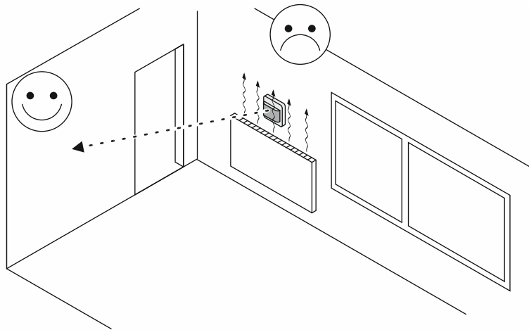
Abb. 35: Störquelle Bewegungsmelder: Bewegte Heizungsluft
