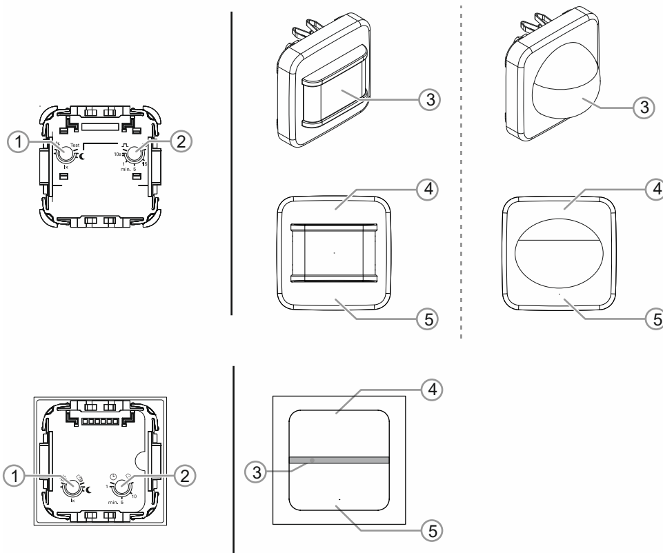
Abb. 18: Bedienelemente
