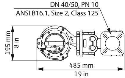
Fig. 2: Bileşenlere ve montaj ölçülerine genel bakış
