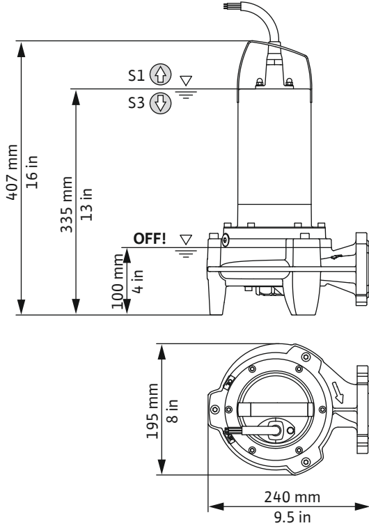
Fig. 3: Montaj ölçüleri
