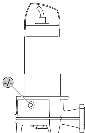
Fig. 8: Камера уплотнений: замена масла
