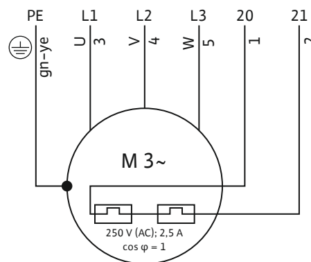
Fig. 7: Schema degli allacciamenti motore 3~
