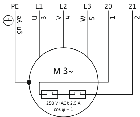
Fig. 7: План на приклучување 3~ мотор
