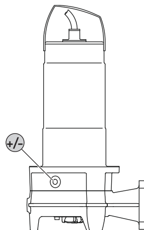
Fig. 8: Заптивна комора: Замена на масло
