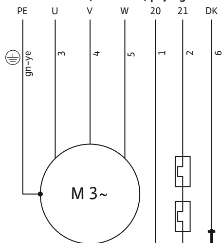
Fig. 7: 3~ variklio prijungimo schema: Tiesioginis paleidimas, bimetalinė juostelė
