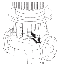
세팅 작업용 포크형 스페이서
