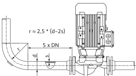
Fig. 13: 펌프 전단 및 후단의 안정화 구간
