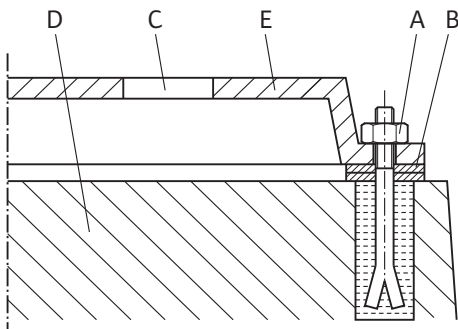
Fig. 12: 기초 나사 연결부 예시
