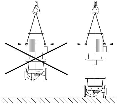
Fig. 2: 모터 운반
