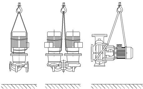
Fig. 1: 펌프 운반
