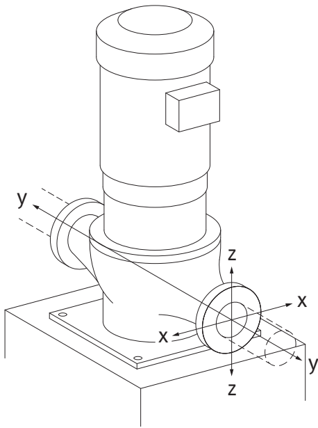
Fig. 7: 로드 케이스 17A, EN ISO 5199, 부칙 B
