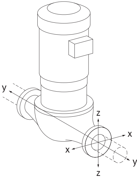
Fig. 6: 로드 케이스 16A, EN ISO 5199, 부칙 B
