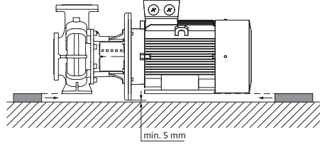
펌프 하우징 및 모터가 지원됨
