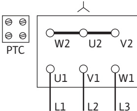
Fig. 15: Y 연결
