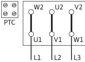
Fig. 14: Δ 결선
