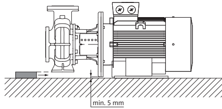
펌프 하우징이 지원됨, 모터가 기초 위에 고정됨
