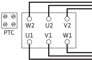
Fig. 16: Y-Δ 연결
