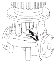
Fig. 17: 포크형 스페이서 장착
