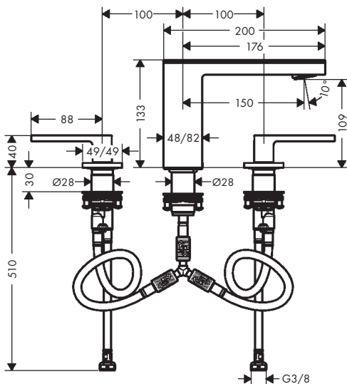
AXOR MyEdition 110 47070XX0 / 47072XX0
