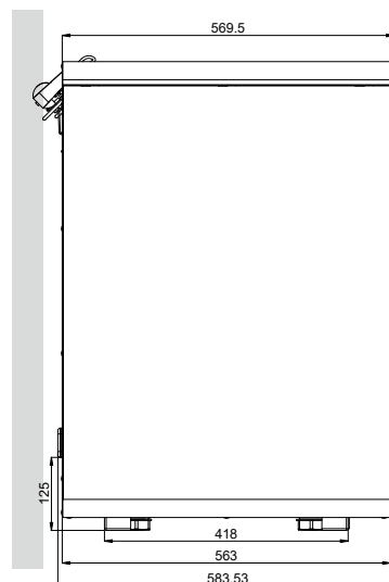
Seitenansicht
