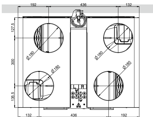
Draufsicht
