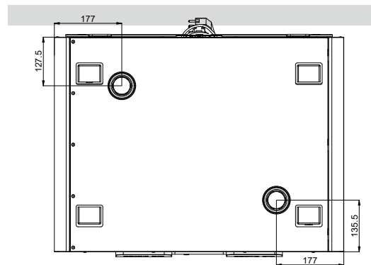
Untersicht
