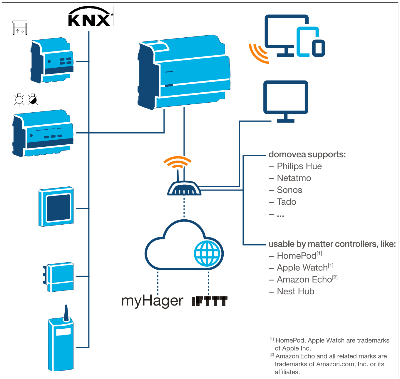
Bild 1: Systemübersicht
