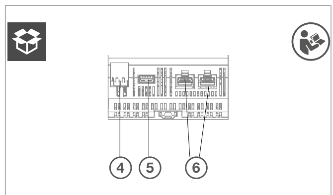
Bild 4: Geräteaufbau - Ansicht von unten auf KNX-, USB- und Ethernet-Schnittstellen
