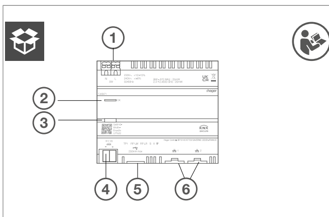
Bild 3: Geräteaufbau - Draufsicht
