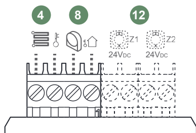
fig. 17 - Aansluitingen Voelers
