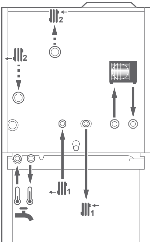
fig. 4 - Hydraulische aansluitingen
