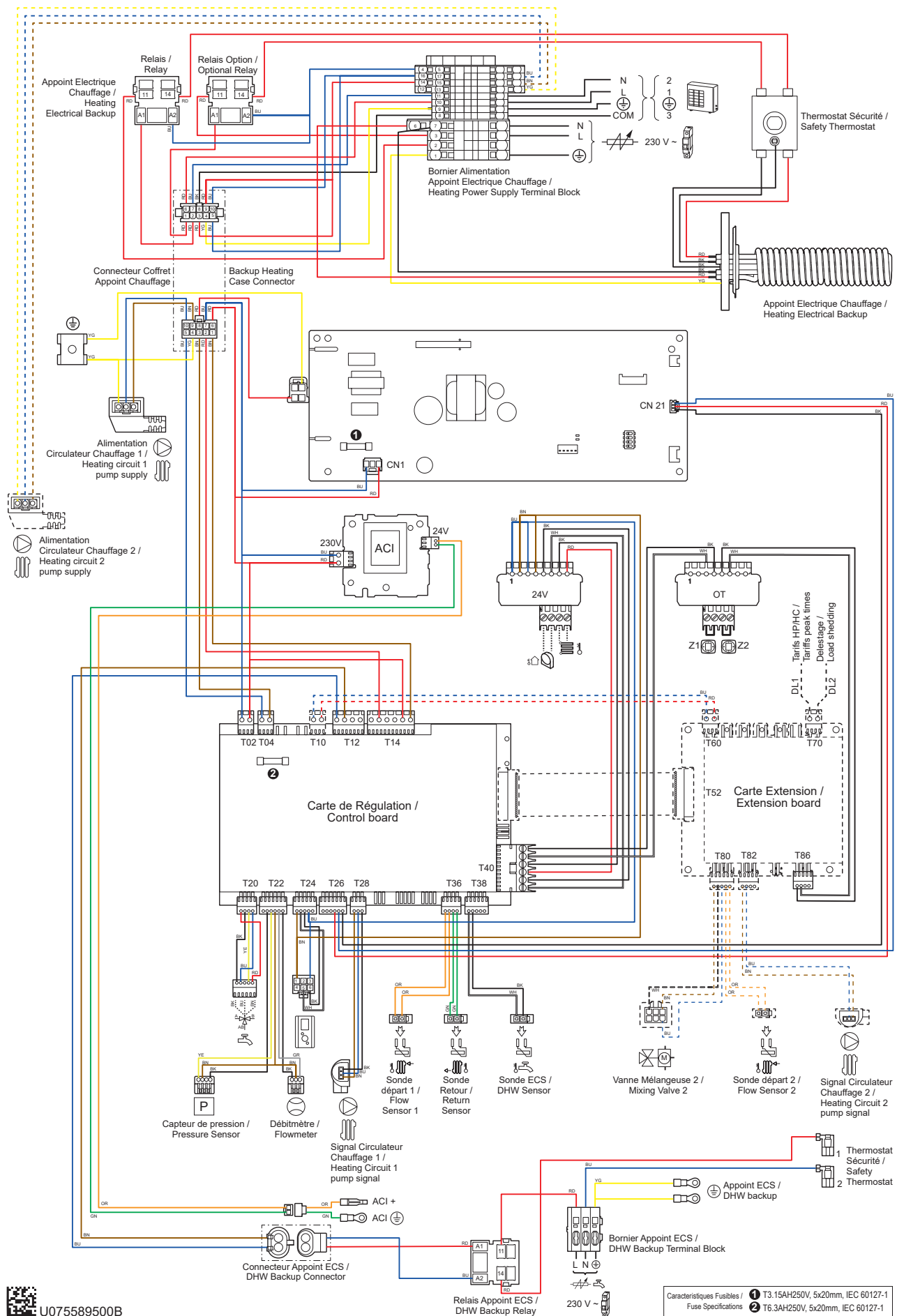
fig. 20 - Elektrische bedrading binneneenheid (m.u.v. aansluitingen installateur)
