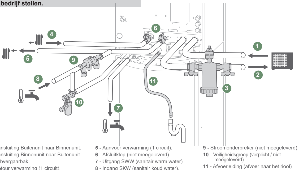
fig. 11 - Aansluitingen
