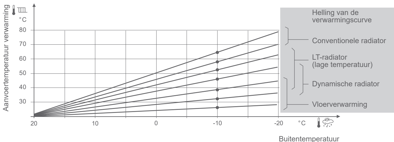
fig. 18 - Helling van de verwarmingscurve
