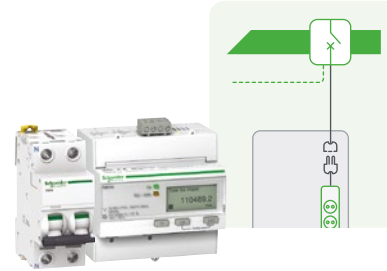
Wired iEM3155
