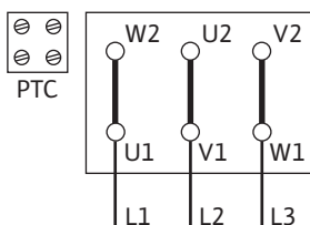
Fig. 14: Δ-lülitus
