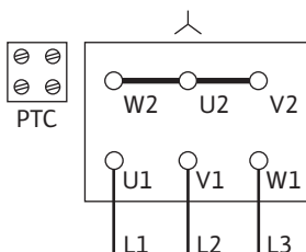
Fig. 15: Y-lülitus
