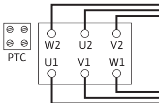
Fig. 16: Y-Δ-lülitus
