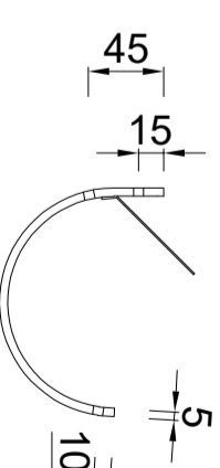
2810004090 RHEINZINK gegalvaniseerde muurbeugel M30 25x5mm tapgat
