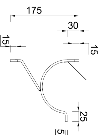
2810004460 RHEINZINK gegalvaniseerde renovatiebeugel M30 25x5mm lip/klang
