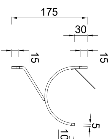
2810004455 RHEINZINK gegalvaniseerde renovatiebeugel M30 25x5mm tapgat
