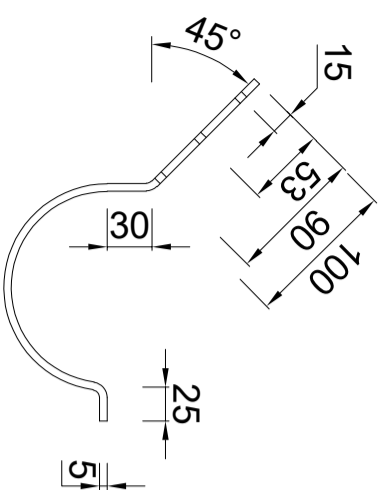
2810000100 RHEINZINK gegalvaniseerde gootbeugel M30 25x5mm lip/klang 45 graden
