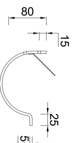
2810003600 RHEINZINK gegalvaniseerde muurbeugel M30 25x5mm lip/klang
