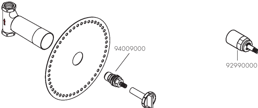
AXOR DN15 (½") 16974180 / 16974187
