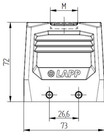
Kabeleingang gerade
