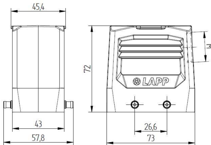
Kabeleingang seitlich
