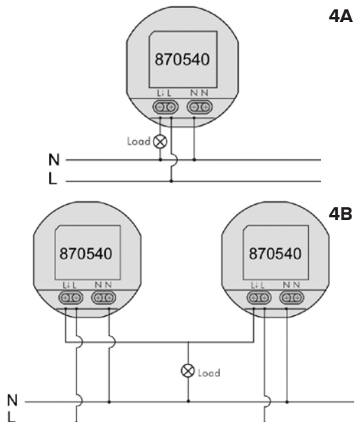
Fig 4: Aansluitschema's
